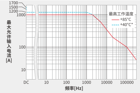
无外部磁场,在导体位置中心定义 * 在最高工作温度+40°C时,允许1500 ADC(连续)和1700 ADC(1分钟)。
